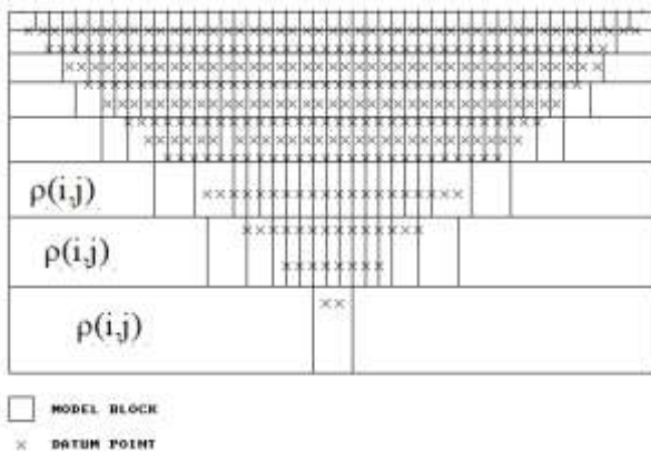
Hình 3: Xấp xỉ mặt cắt tuyến đo bằng các khối hình chữ nhật có điện trở suất \rho(i,j)
