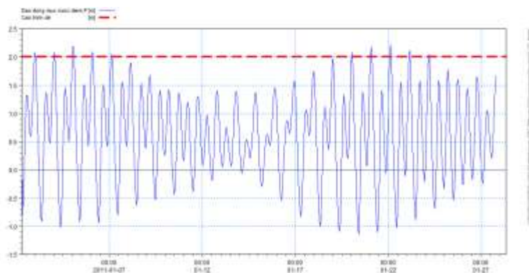
Hình 6: Vị trí điểm trích xuất dòng chảy - cách đê 50m (trái) và Biểu đồ so sánh dao động mực nước điểm P với cao trình đỉnh đê
