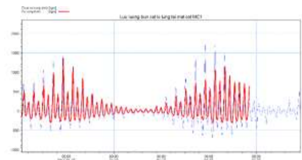
Hình 11: So sánh lưu lượng bùn cát dọc bờ phương án chưa có công trình và có công trình
