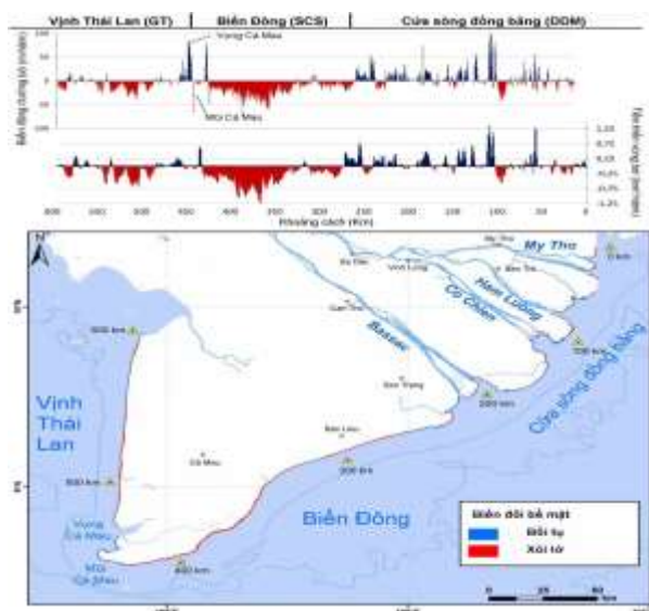
Hình 1: Hình trên: Đồ thị biểu diễn tốc độ biến đổi đường bờ (m/năm, sai số \pm 0.5 m/năm) và diện tích vùng bờ (km 2 /năm, sai số \pm 0.005 km 2 /năm) vùng Đồng bằng sông Cửu Long giai đoạn 2003-2011/2012. Hình dưới: Bản đồ xói lở, bồi tụ tại 3 đoạn bờ ĐBSCL: Tốc độ xói lở dọc theo đoạn bờ Biển Đông tăng dần về phía tây nam cùng với khoảng cách xa dần các cửa sông. [11]
