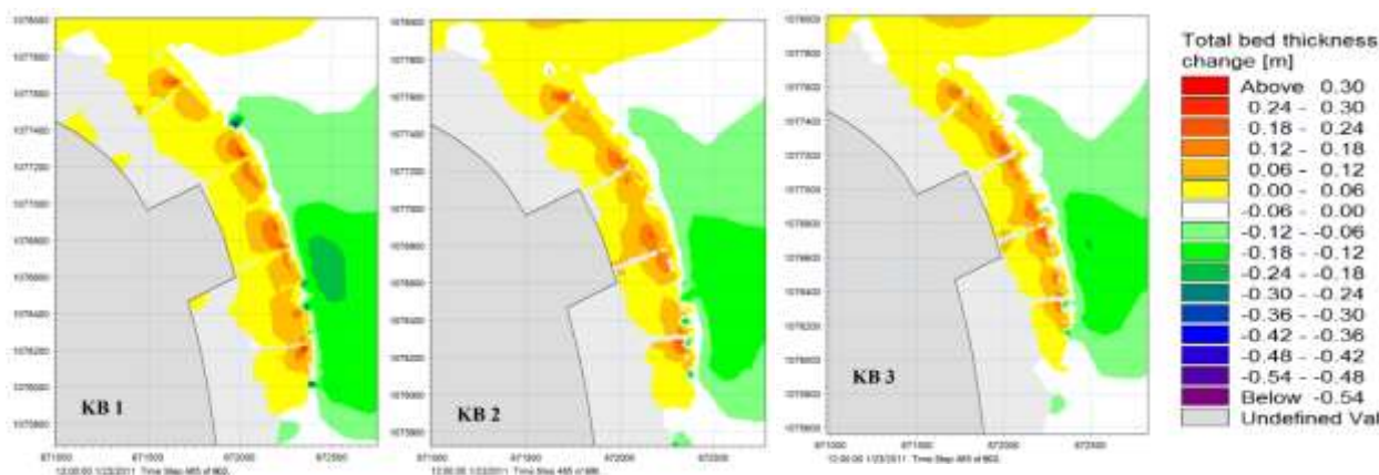
Hình 13: Diễn biến bồi xói khu vực bờ biển xã Hiệp Thạnh phương án có công trình sau 1 tháng tính toán (1-23/1/2011, mùa gió đông bắc)
