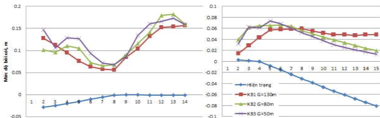
Hình 12: Mức độ bồi tụ tại mặt cắt 3 (trái) và mặt cắt 4 (phải) sau 1 tháng
