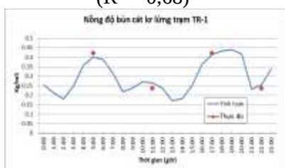
Kiểm tra nồng độ bùn cát lơ lửng tại trạm TR-1
