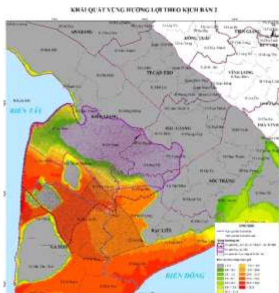
Hình 6: Kết quả mô phỏng diễn biến xâm nhập mặn trong mùa khô sau 12 ngày vận hành hệ thống công trình CL-CB và công
