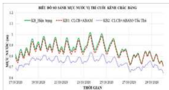
Hình 15: Biểu đồ so sánh mực nước vị trí cuối kênh Chắc Băng
