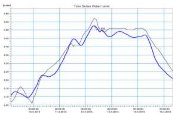
Hình 12: Mức nước tính toán và thực đo tại hạ lưu đập Thạch Nham 2013
