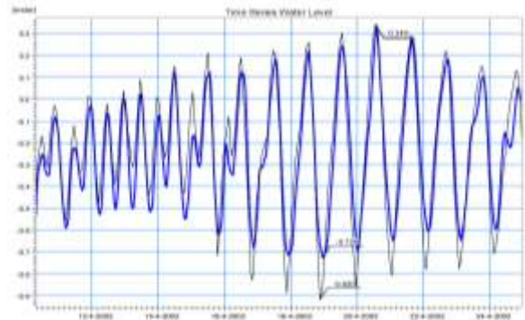
Hình 8: Mực nước mô phỏng và thực đo tại cửa Cổ Lũy 2002
