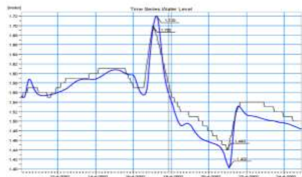
Hình 10: Mực nước mô phỏng và thực đo tại trạm Trà Khúc 2002
