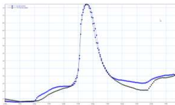
Hình 14: So sánh kết quả mô phỏng và thực đo tại trạm thủy văn Trà Khúc (Đường màu xanh là kết quả mô phỏng, đường màu đen là số liệu thực đo)
