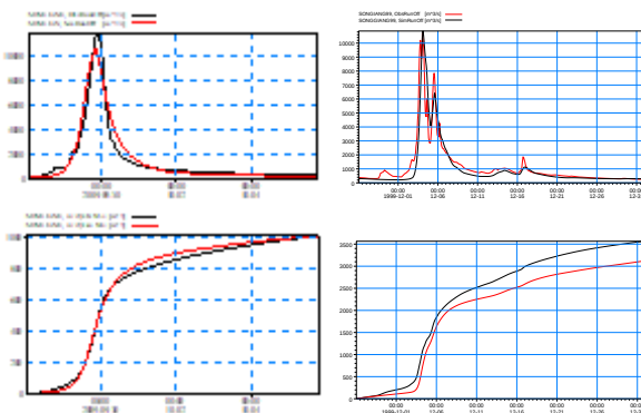
Hình 7: Kết quả hiệu chỉnh, kiểm định mô hình mưa dòng chảy
