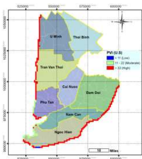
Hình 14a: Bản đồ chỉ số tổn thương vật lý vùng bờ theo thang điểm 3 cấp (PCVI)
