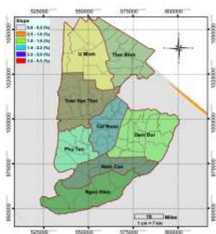
Hình 6: Bản đồ độ dốc bờ biển Cà Mau
