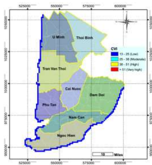
Hình 18b: Bản đồ chỉ số tổn thương tổng hợp vùng bờ theo thang điểm 5 cấp (CVI)
