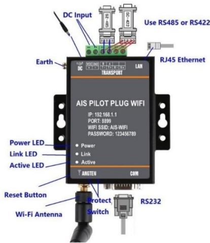
Hình 3. Cấu hình bộ chuyển đổi dữ liệu AIS
