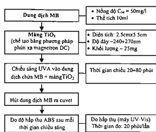
Hình 4. Sơ đồ mô tả quy trình đo quang xúc tác sử dụng MB cho màng TiO 2 .
