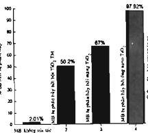
Hình 11. Sự phân hủy MB của các vật liệu nano TiO 2 ở thời gian chiếu sáng UVA 80 phút.
