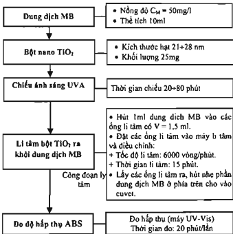
Hình 6. Sơ đồ mô tả quy trình đo quang xúc tác sử dụng MB cho bột nano TiO 2 .
