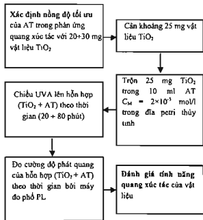
Hình 7. Sơ đồ mô tả quy trình đo quang xúc tác của vật liệu nano TiO 2 bằng axit terephthalic.
