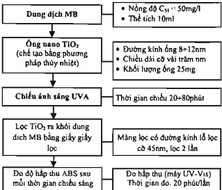
Hình 5. Sơ đồ mô tả quy trình đo quang xúc tác sử dụng MB cho ống nano TiO 2 .
