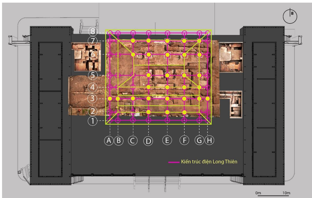
Hình 12. Mặt bằng kiến trúc điện Long Thiên thời Nguyễn
