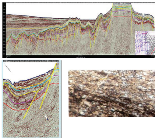
Hình 1: phức tập S 1 - Oligocen sớm (E 3 1 ). Bột kết hạt nhỏ, bị nén ép và phiến hoá mạnh, nền chủ là xi măng canxit (C) và vật chất hữu cơ tướng sét đầm lầy ven biển thuộc hệ thống trầm tích biển tiến (TST). Mẫu ở độ sâu 2705 m; E 3 1 ; tuổi Oligocen; N + ; x125 (PV-94-2X) bề Tư Chính - Vũng Mây
