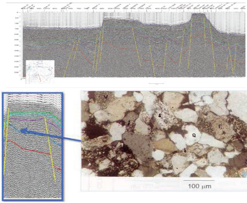
Hình 3: phức tập S_3 (N_1^1) khu vực Tư Chính - Vũng Mây. Cát kết với thành phần chủ yếu là thạch anh (Q), K-felspat (F), mảnh đá phun trào (V) chọn lọc, mài tròn tốt, phiến sét (S), ít mica (xanh). Xi măng sét lấp đầy lỗ hổng giữa hạt đặc trưng tương trầm tích sóng (LST). Mẫu ở độ sâu 2320 m; N_1^1 ; PV-94-2X; N^+ ; x125 bề Tư Chính - Vũng Mây
