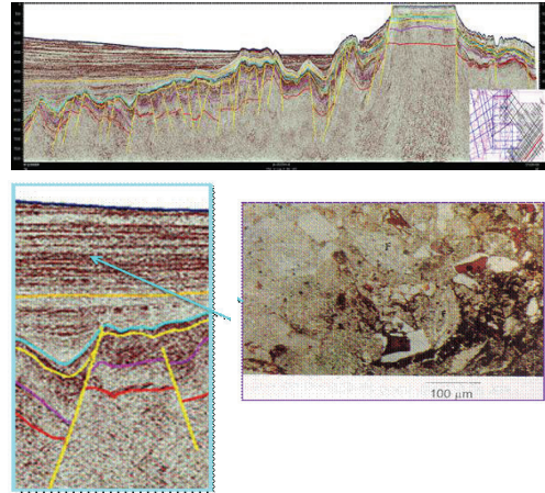
Hình 7: phức tập S 6 (N 2 -Q). Lát mỏng chỉ ra ranh giới giữa cát kết thạch anh xi măng canxit vi hạt với cát kết lục nguyên chứa vụn vỏ sinh vật. Đá thuộc tướng bãi triều ven biển có sóng hoạt động mạnh thành tạo trong pha biển thoái của biển thấp (LST) (amr LST). Mẫu ở độ sâu 1160 m, N + , x125
