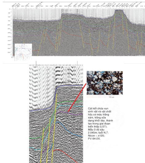
Hình 4: phức tập S_4 (N_1^2) giai đoạn biển thấp (LST)
