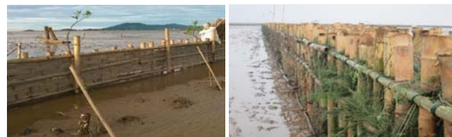
Hình 2: kết cấu tường mềm đơn Hình 3: kết cấu tường mềm kép
