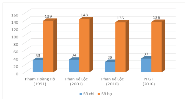
Biểu đồ 1. Số lượng các họ và chi nhóm Khuyết thực vật ở Việt Nam theo các quan điểm khác nhau.
