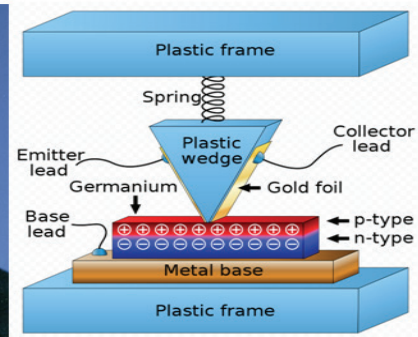
Hình 2. Cấu trúc của transistor tiếp điểm mà Bardeen and Brattain đã ghi chép vào sổ tay thí nghiệm ngày 16/12/1947 (nguồn: Google Images).
