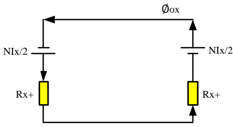
H. 11 Mạch từ phần ngoài không có nam châm vĩnh cửu
