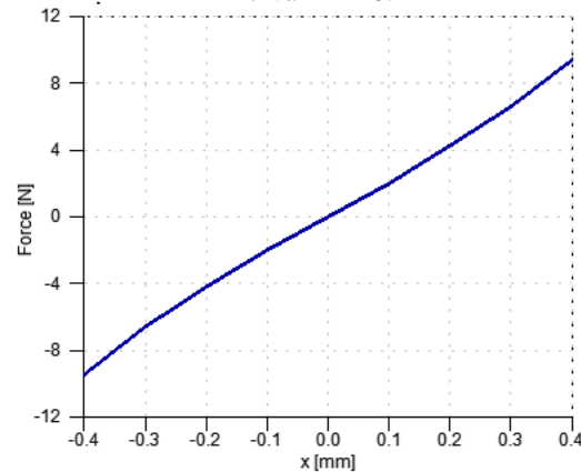
H. 7 Lực hướng tâm biến đổi theo độ dịch chuyển rotor
