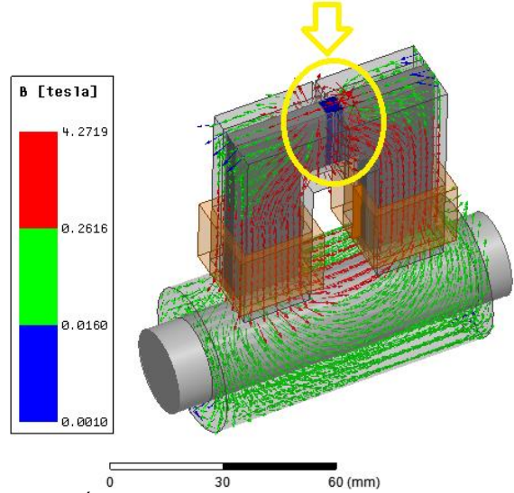
H. 6 Kết quả mô phỏng FEM của HBM có khe hở không khí phụ. Thông quan việc mô phỏng này, kết quả phân tích lực theo độ dịch chuyển của rotor và theo dòng điều khiển của một cực từ thu được như Hình 7 và Hình 8.
