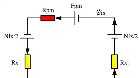
H. 10 Mạch từ phần giữa có nam châm vĩnh cửu
