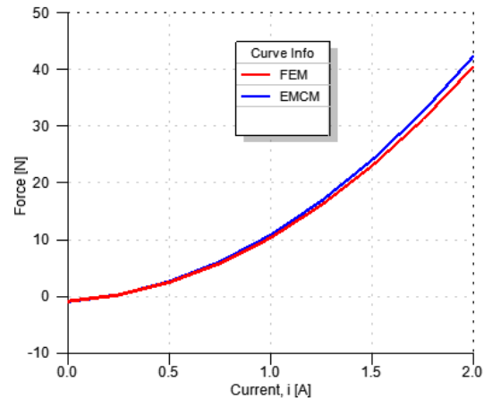
H. 13 Lực hút của cực từ phía trên lên rotor ứng với x = -0.4\text{mm}
