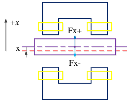
H. 3 Rotor dịch chuyển lên một khoảng x theo chiều (+x)
