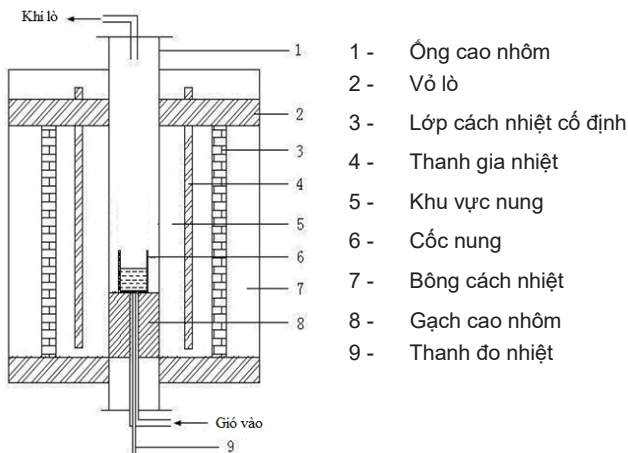
Hình 2. Cấu tạo lò giồng
