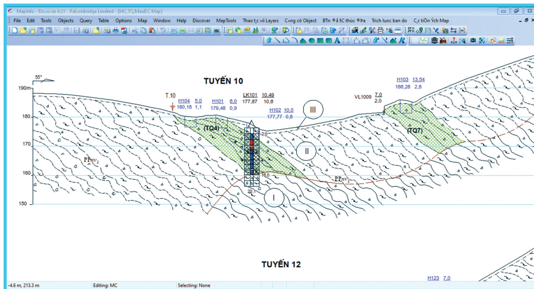
Hình 2. Đới phong hóa chứa quặng vermiculite khu khu Phố Ràng (Hiệu chỉnh từ Liên đoàn Địa chất Xạ - Hiếm, 2017)
