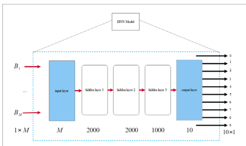
Hình 9. DNN model
