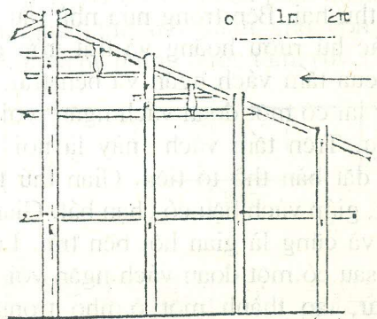
B.v 6: Kiểu vì kèo cổ truyền nhà người Tày, Nùng
