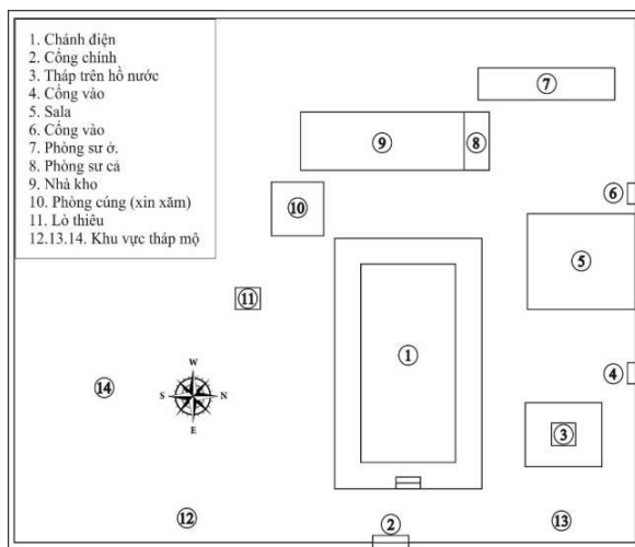
Hình 1. Mặt bằng chùa Prây – Veng (Huyện Tri Tôn) Nguồn: Tác giả
