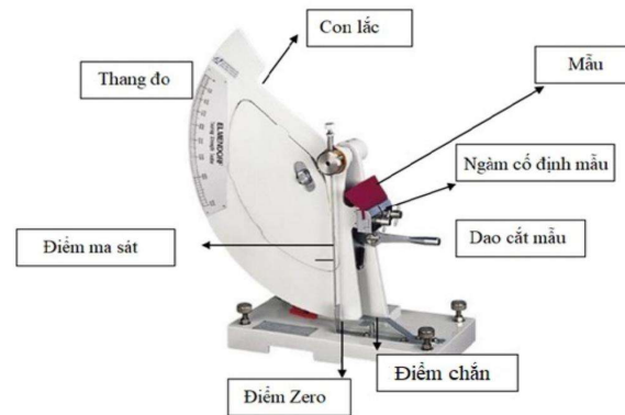
Hình 2.1: Hình thiết bị xé rách
