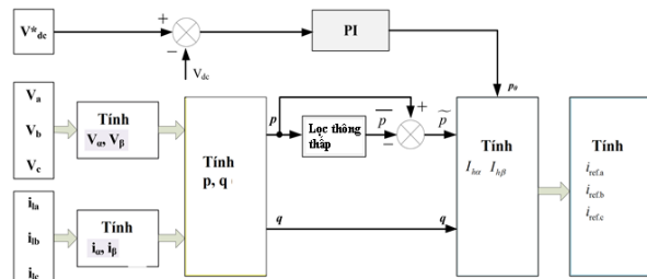
Hình 2.2. Cấu trúc của bộ xác định dòng điện bù
