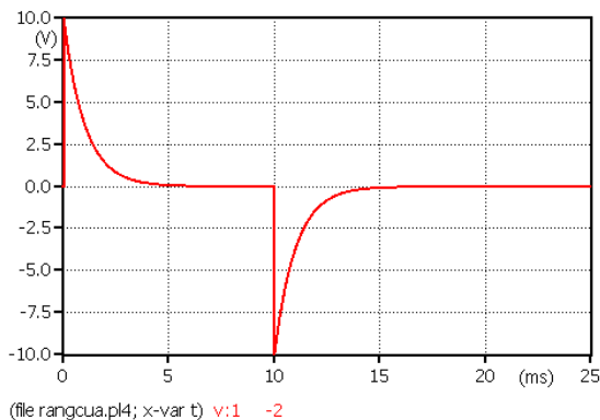
Hình 2.6. Kết quả mô phỏng đáp ứng của mạch R-C với nguồn xung chu kỳ: Xung nguồn và điện áp trên tụ trong ba trường hợp: C = 10 \mu F , C = 100 \mu F , C = 1000 \mu F .
