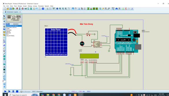
Hình 2.2: Mô phỏng mạch điện trên phần mềm Protues
