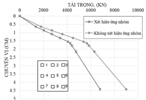
Hình 16. Ứng xử đài cọc chịu tải đứng
