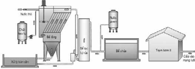
Hình 1. Sơ đồ dây chuyền công nghệ xử lý nước mặt với bể lắng lamen, bể lọc vật liệu
