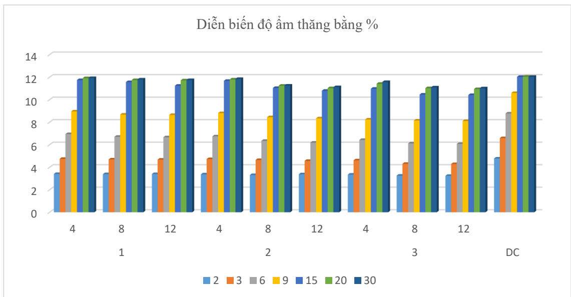
Hình 6. Biểu đồ quan hệ giữa nồng độ và thời gian xử lý nano ZnO với độ ẩm thẳng bằng
