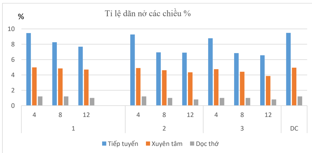
Hình 5. Biểu đồ quan hệ giữa nồng độ và thời gian xử lý nano ZnO với độ dẫn nở
