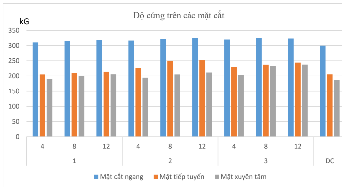
Hình 7. Độ cứng trên 3 mặt cắt (ngang, tiếp tuyến, xuyên tâm)
