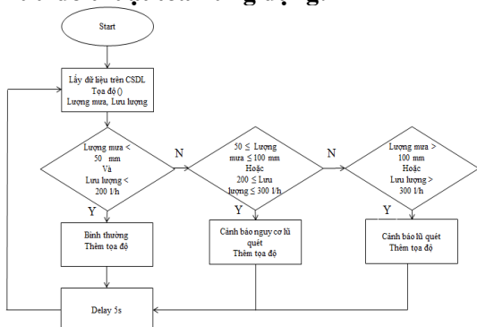
Hình 10. Lưu đồ thuật toán ứng dụng
