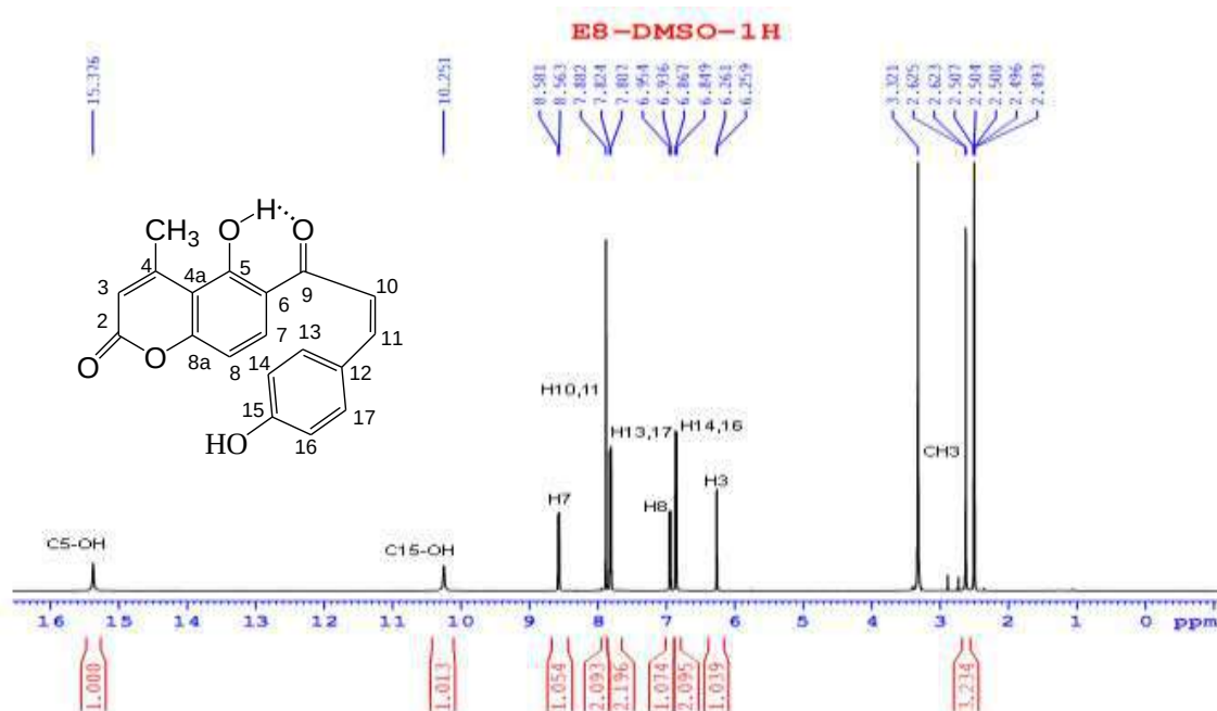
Hình 2. Phổ ^1\text{H} NMR của \text{I}_3
