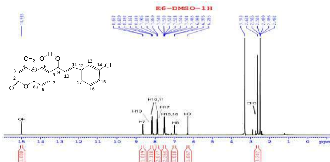
Hình 1. Phổ ^1\text{H} NMR của \text{I}_1
