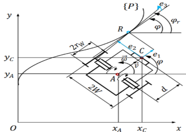
Hình 1. Mô hình robot tự hành ba bánh
