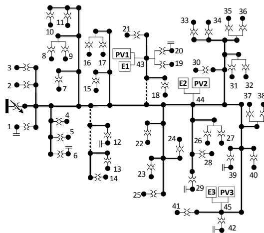
Hình 4. Cấu trúc LĐPP đề xuất tính toán [12]
