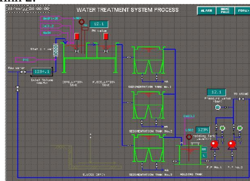
Hình 3. Giao diện quá trình hệ thống xử lý nước
