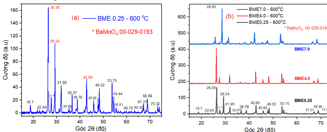
Hình 2. Giản đồ XRD của các \text{BaMoO}_4@x\text{Eu}^{3+} : (a) x = 0,25 ; (b) x = 0,25 ; 4,0 và 7,0 nung ở 600^\circ\text{C}
