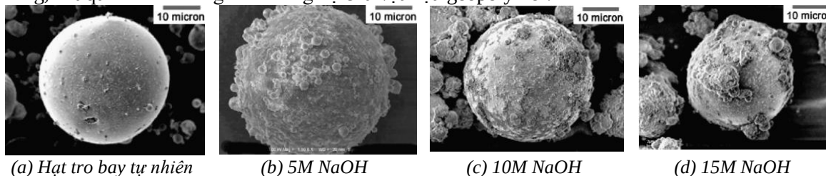
(a) Hạt tro bay tự nhiên (b) 5M NaOH (c) 10M NaOH (d) 15M NaOH Hình 19. Kết quả phân tích bề mặt hạt tro bay ở các trạng thái khác nhau: (a) tự nhiên, (b) trong dung dịch NaOH 5M, (c) NaOH 10 M, và (d) NaOH 15M [52]
