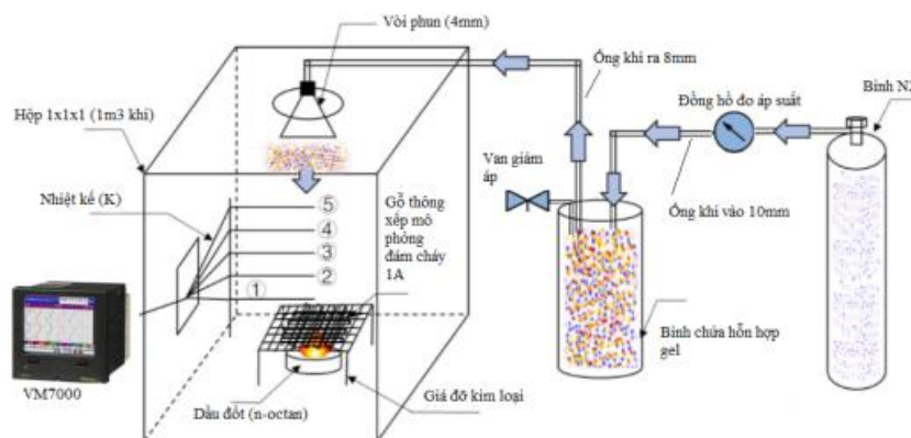
Hệ thí nghiệm chữa cháy quy mô nhỏ (hình 1) được xây dựng theo các tiêu chuẩn về thử nghiệm chữa cháy như: GB4066-2017, GB 17835-2008, ISO 7202-2012, NFPA 17, ANSI/UL 299 đã được mô tả trong các công trình trước đây [3], [13].
