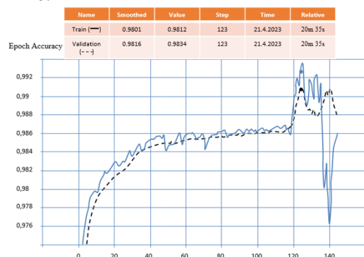
Hình 5. Biểu đồ Accuracy - LSTM – CICIDS2017 theo số Step
