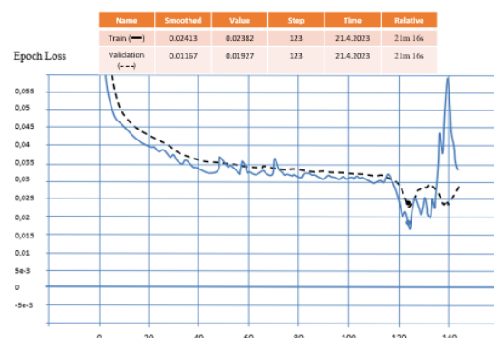
Hình 6. Biểu đồ Loss – LSTM – CICIDS2017 theo số Step
