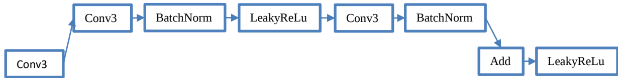
Hình 5. Kiến trúc của một khối ResBlock1D
