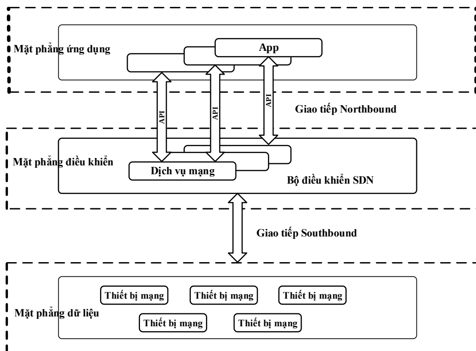
Hình 1. Kiến trúc của SDN
