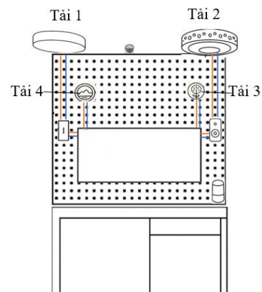
Hình 6. Sơ đồ kết nối công tắc Tuya đến phụ tải
