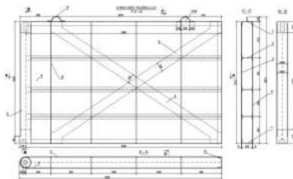
Hình 5: Kết cấu cửa van tự động
