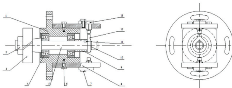
Hình 4. Mặt cắt bộ tạo xung đánh lửa cải tạo từ bộ dẫn động bơm cao áp
