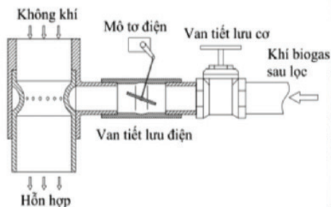
Hình 6. Bộ hòa trộn hỗn hợp khí
