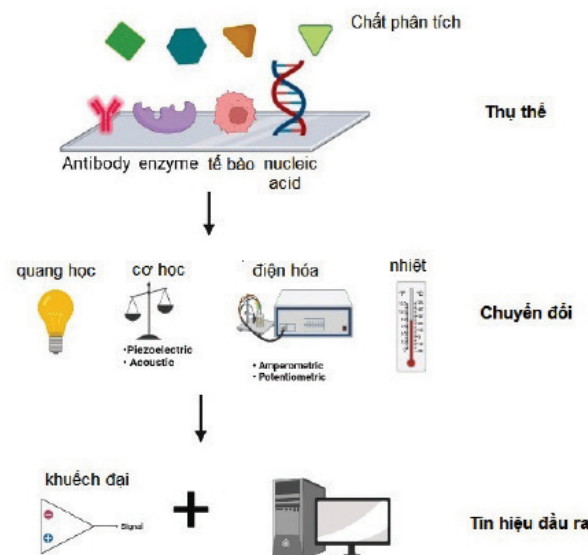
Hình 1. Các thành phần điển hình của một cảm biến sinh học
