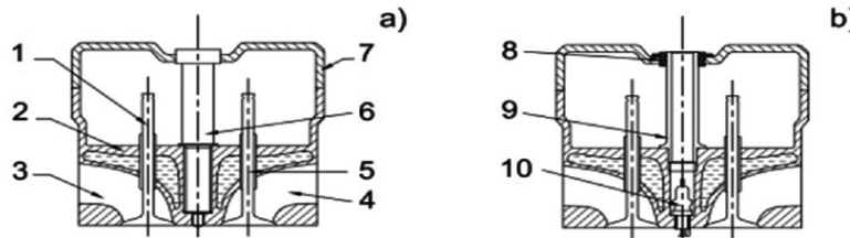
Hình 2. Mặt cắt vị trí lắp đặt vòi phun và bugi 1- Xupap nạp 4- Cửa xả 6- Vòi phun 9- Ống lót 2- Nắp máy 5- Xupap xả 7- Nắp che 10- Bugi 3- Cửa nạp 8- Phốt chặn dầu
