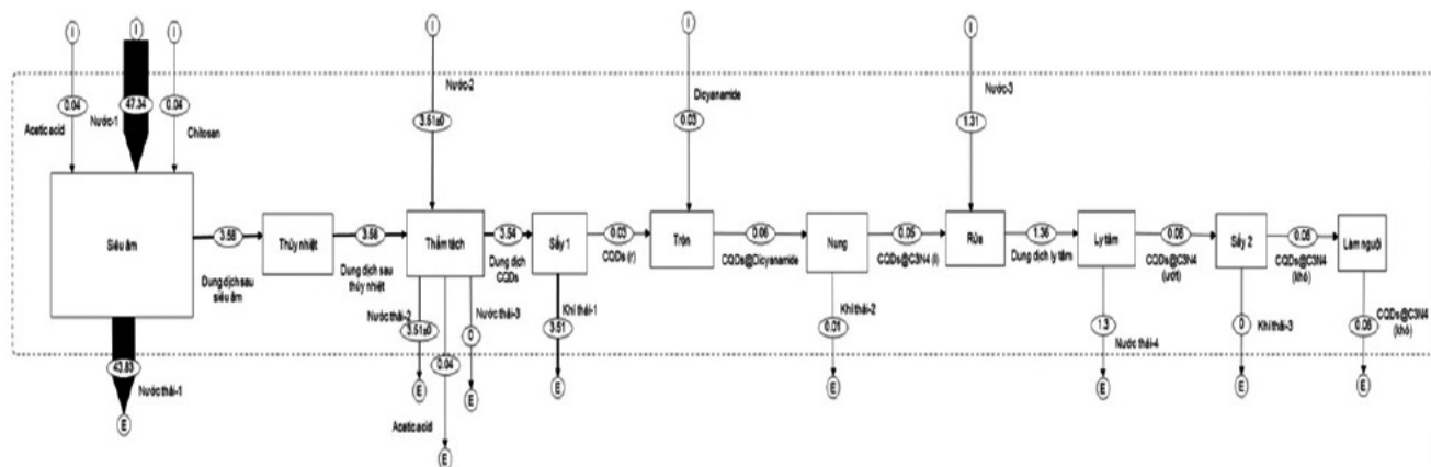
Hình 2. Sơ đồ dòng vật chất trong quá trình tổng hợp vật liệu C_3N_4 mang CQDs
