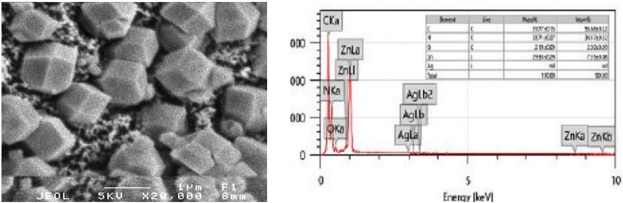
Hình 4. Hình ảnh AgNPs/ZIF-8 được chụp qua (a) SEM và phân tích (b) EDS
