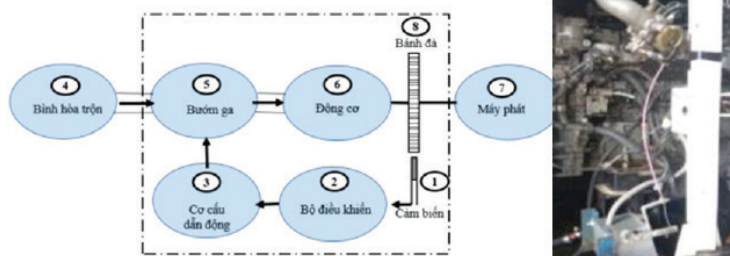
Hình 7. Bộ ổn định tốc độ
