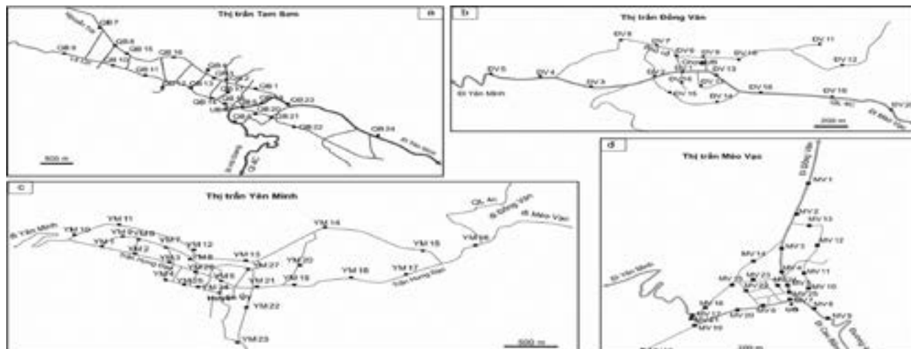
▲ Hình 3. Sơ đồ vị trí các điểm đo nồng độ radon trong không khí tại các khu đô thị: a) thị trấn Tam Sơn, huyện Quản Bạ, b) thị trấn Đông Văn, huyện Đông Văn, c) thị trấn Yên Minh, huyện Yên Minh, d) thị trấn Mèo Vạc, huyện Mèo Vạc
