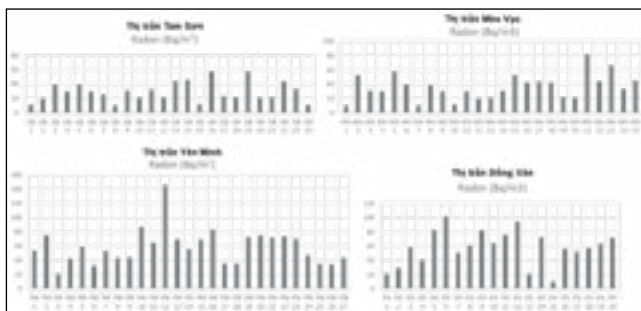
▲ Hình 4. Biểu đồ phân bố nồng độ radon trong không khí tại các khu đô thị vùng Cao nguyên đá Đồng Văn
