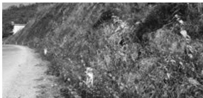
▲ Hình 6. Điểm đo YM12 có nồng độ radon cao 145 Bq/m 3
