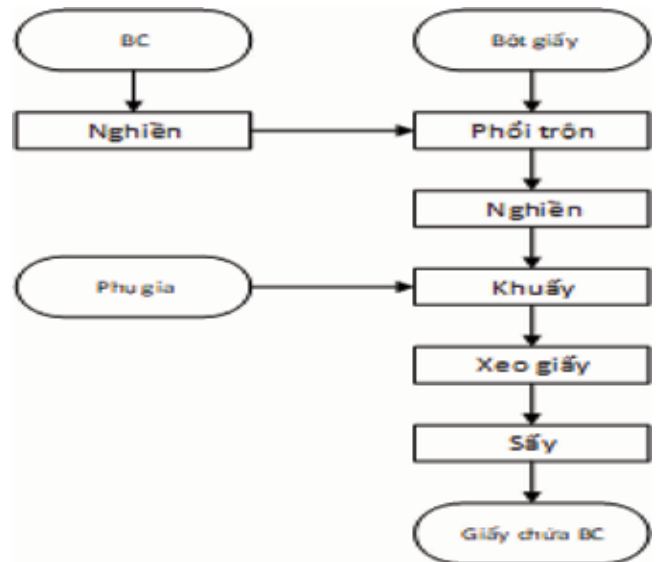
▲ Hình 7. Quy trình xeo giấy chứa BC
