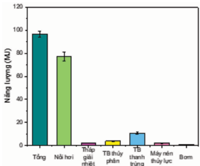
▲ Hình 9. Mức năng lượng trung bình cho 1 m 3 sản xuất BC
