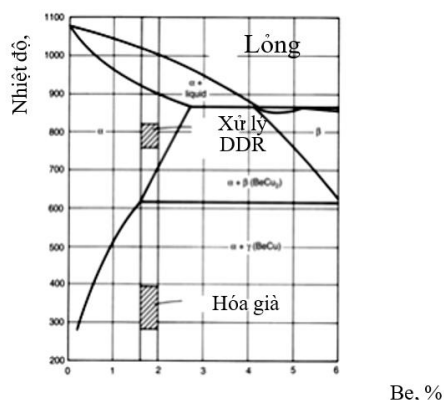
Hình 1. Thành phần và khoảng nhiệt độ xử lý nhiệt
