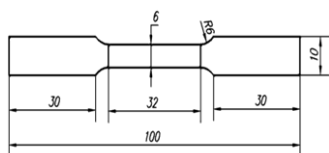
Hình 3. Mẫu đo bền kéo
