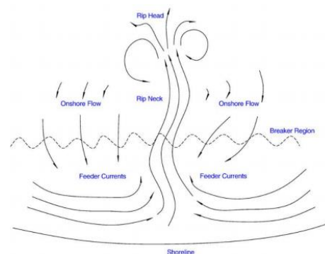
Hình 1. Sơ đồ hoàn lưu dòng chảy xiết
