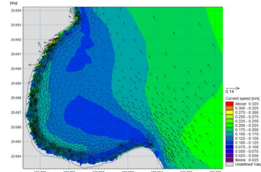
Hình 11. Trường dòng chảy xiết tháng 9 pha triều lên
