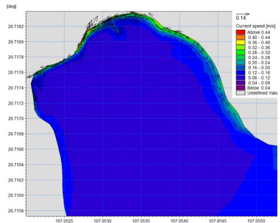
Hình 19. Dòng chảy xiết trong pha triều lên tháng 8
