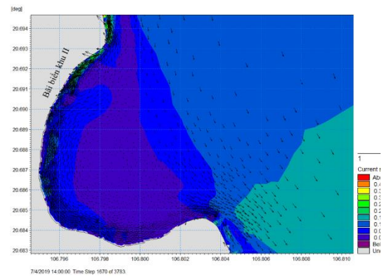
Hình 6. Dòng chảy xiết khi triều rút gió mùa mạnh
