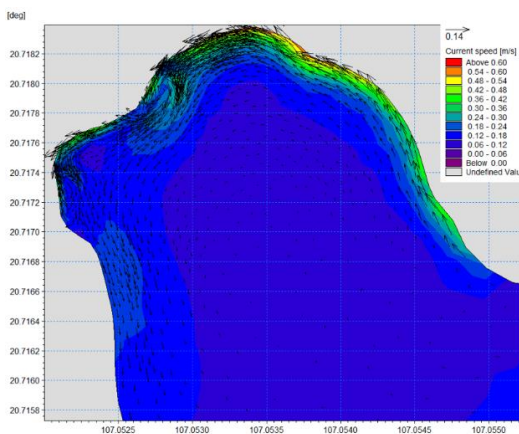
Hình 17. Dòng chảy xiết trong pha triều rút tháng 6
