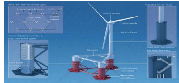
Hình 2. Mô hình WindFloat Atlantic (PPI)
