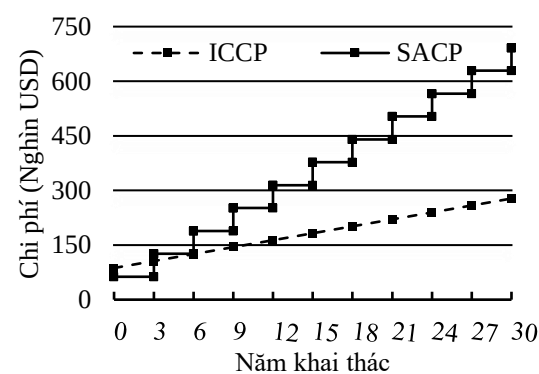
Hình 9. Chi phí lắp đặt và vận hành hệ thống bảo vệ ăn mòn tàu Vosco Sky
