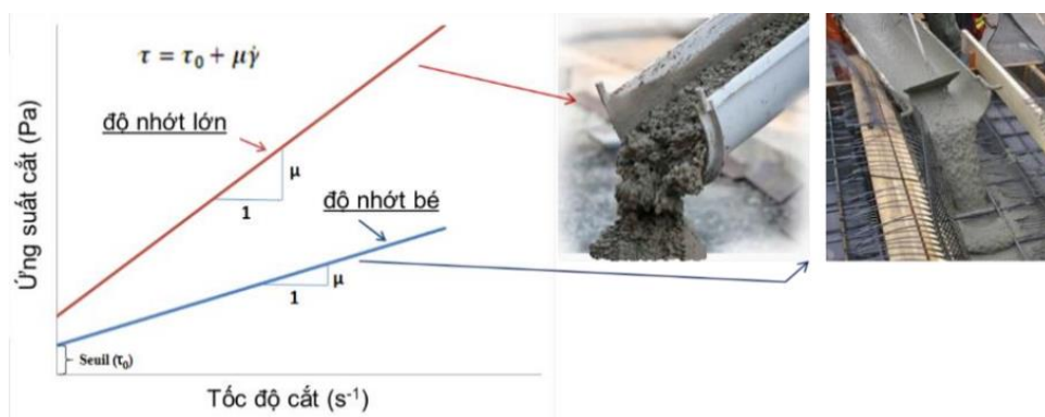
Hình 1: Các trạng thái lưu biến của vữa bê tông tươi [6]
